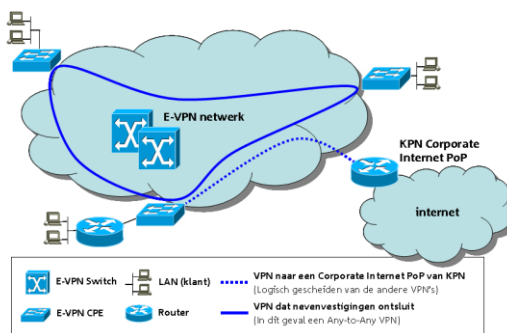
Figuur 5: Corporate Internet en Ethernet VPN
