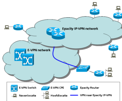
Figuur 6: One en Epacity IP-VPN en Ethernet VPN
